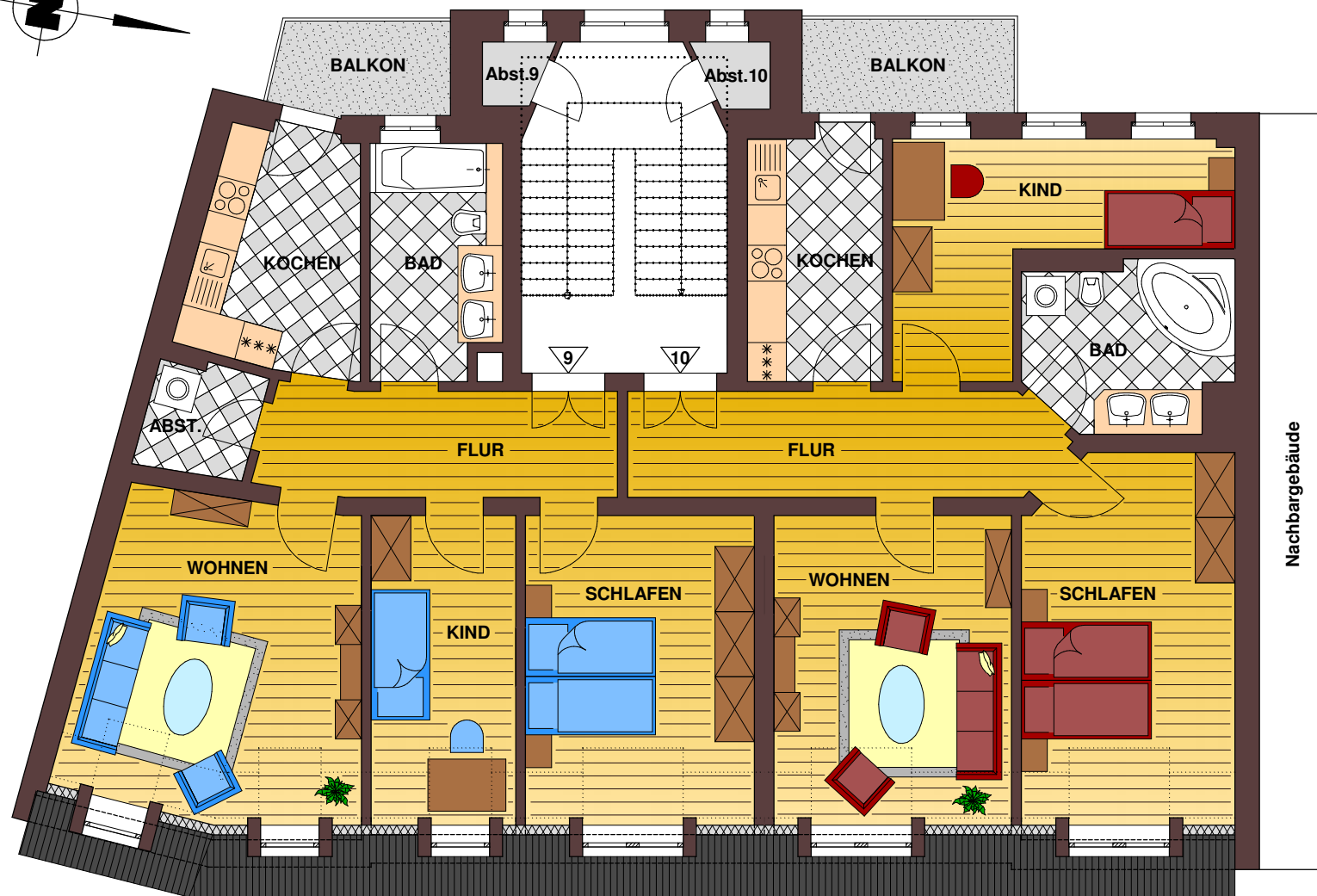
Zusammenstellung der Flächen Dachgeschoss
